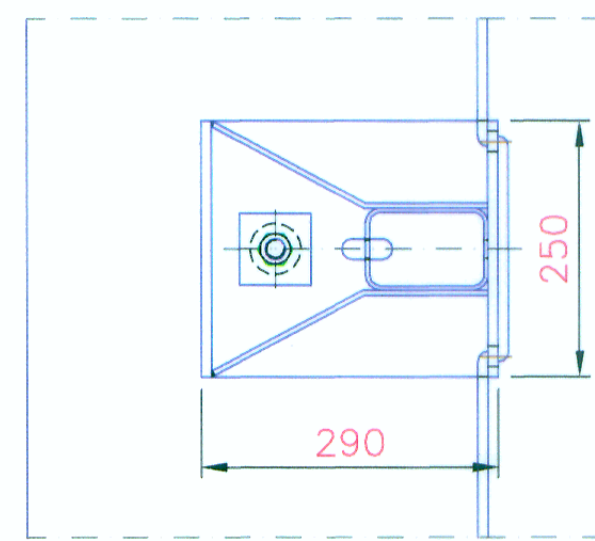
SECCIÓN A-A
