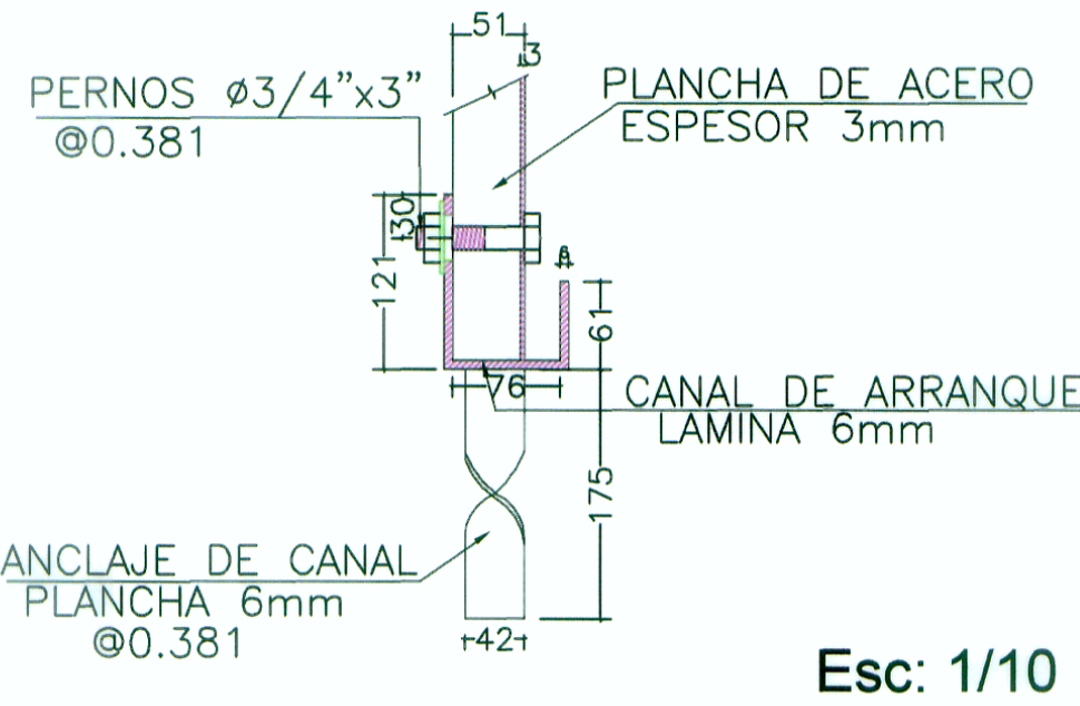
DETALLE " A "
