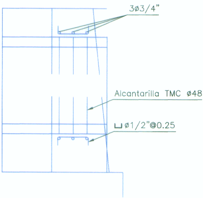
SECCIÓN A-A
