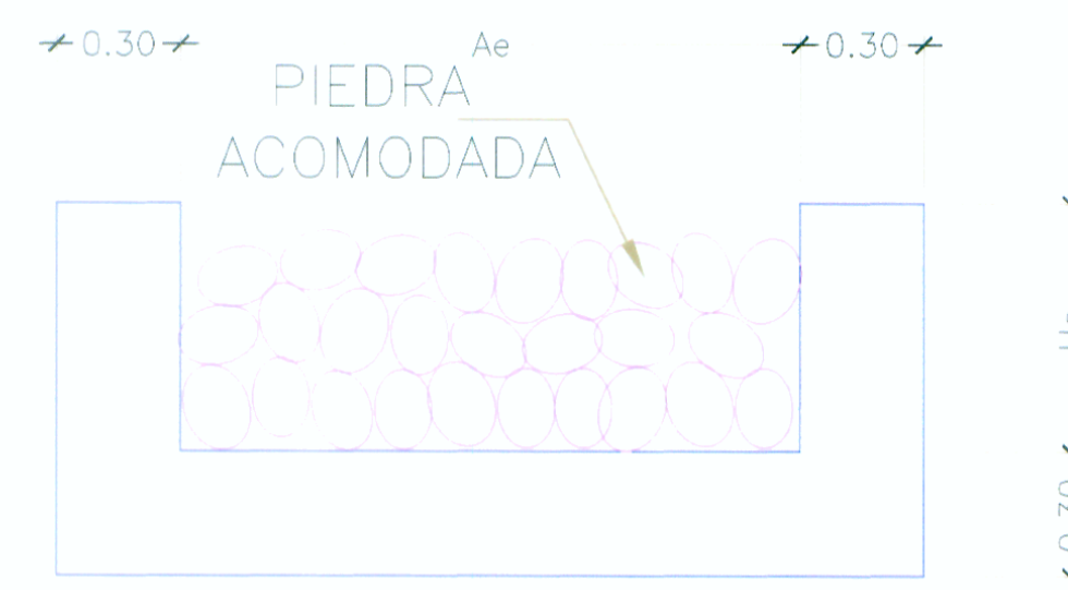
CORTE B-B ESC.1/20
