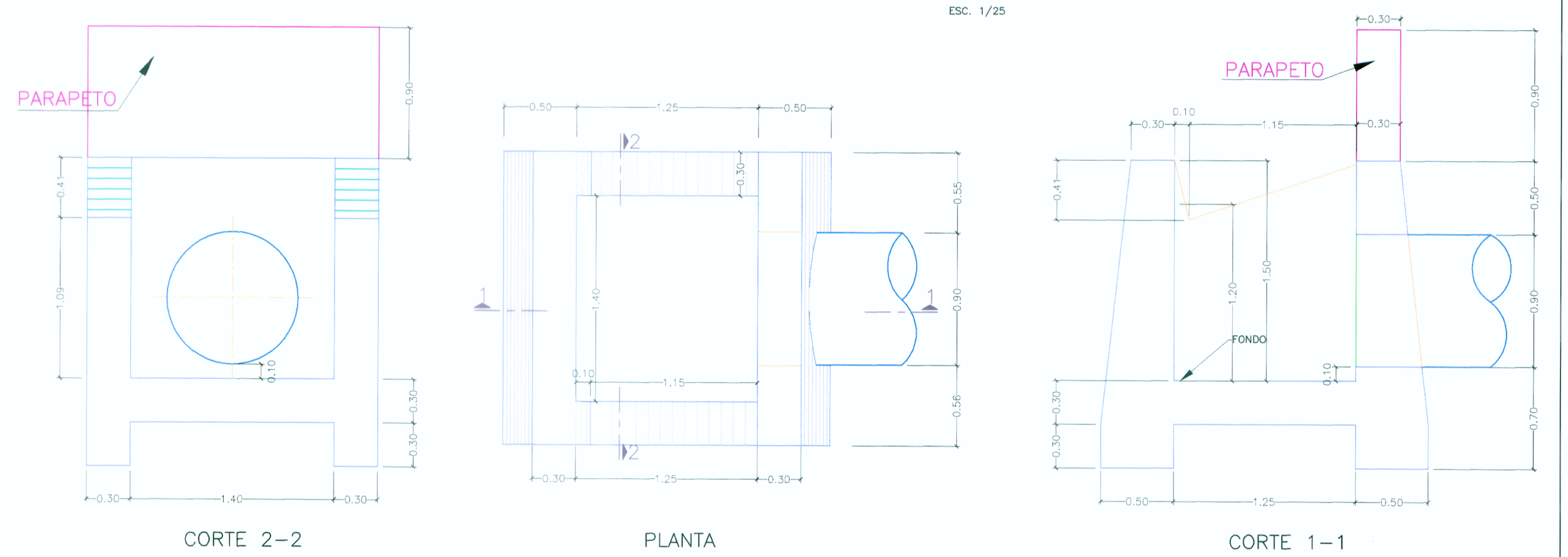
CAJA RECEPTORA TIPO 2 Ø 36" ESC. 1/25
