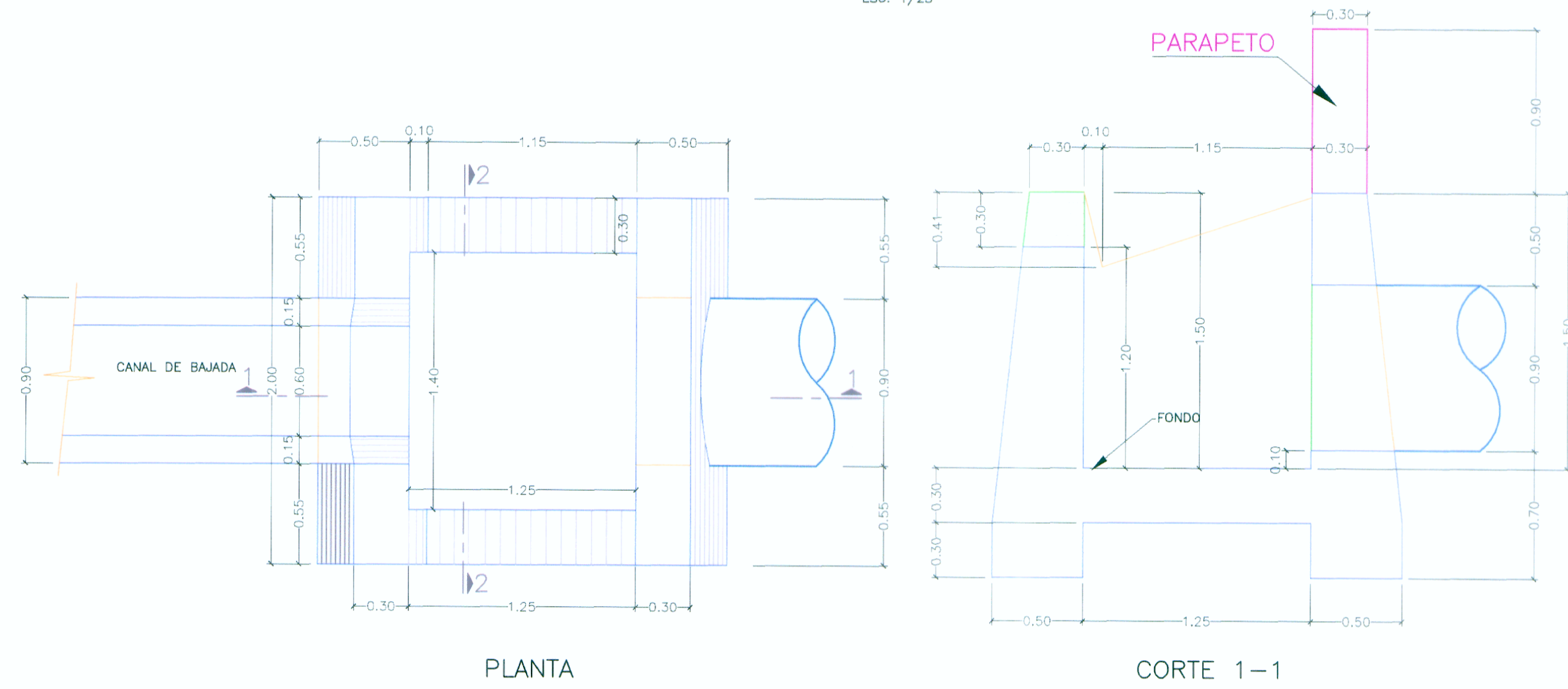
CAJA RECEPTORA TIPO 1 Ø 36" ESC. 1/25
