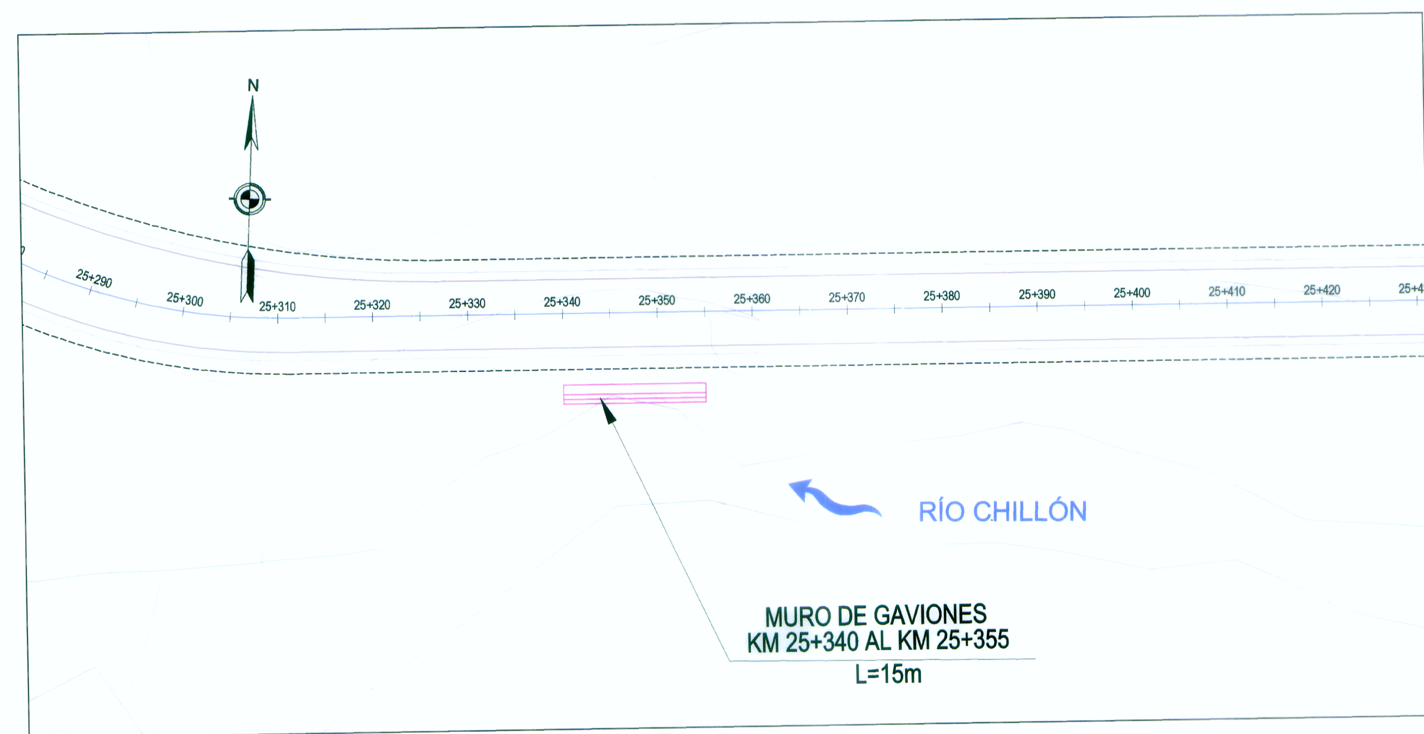
PLANTA
