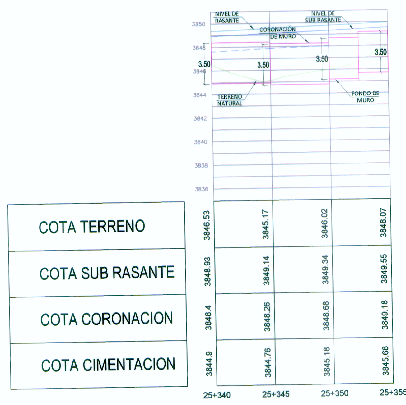
Muro Gavión 25+340 - 25+355
