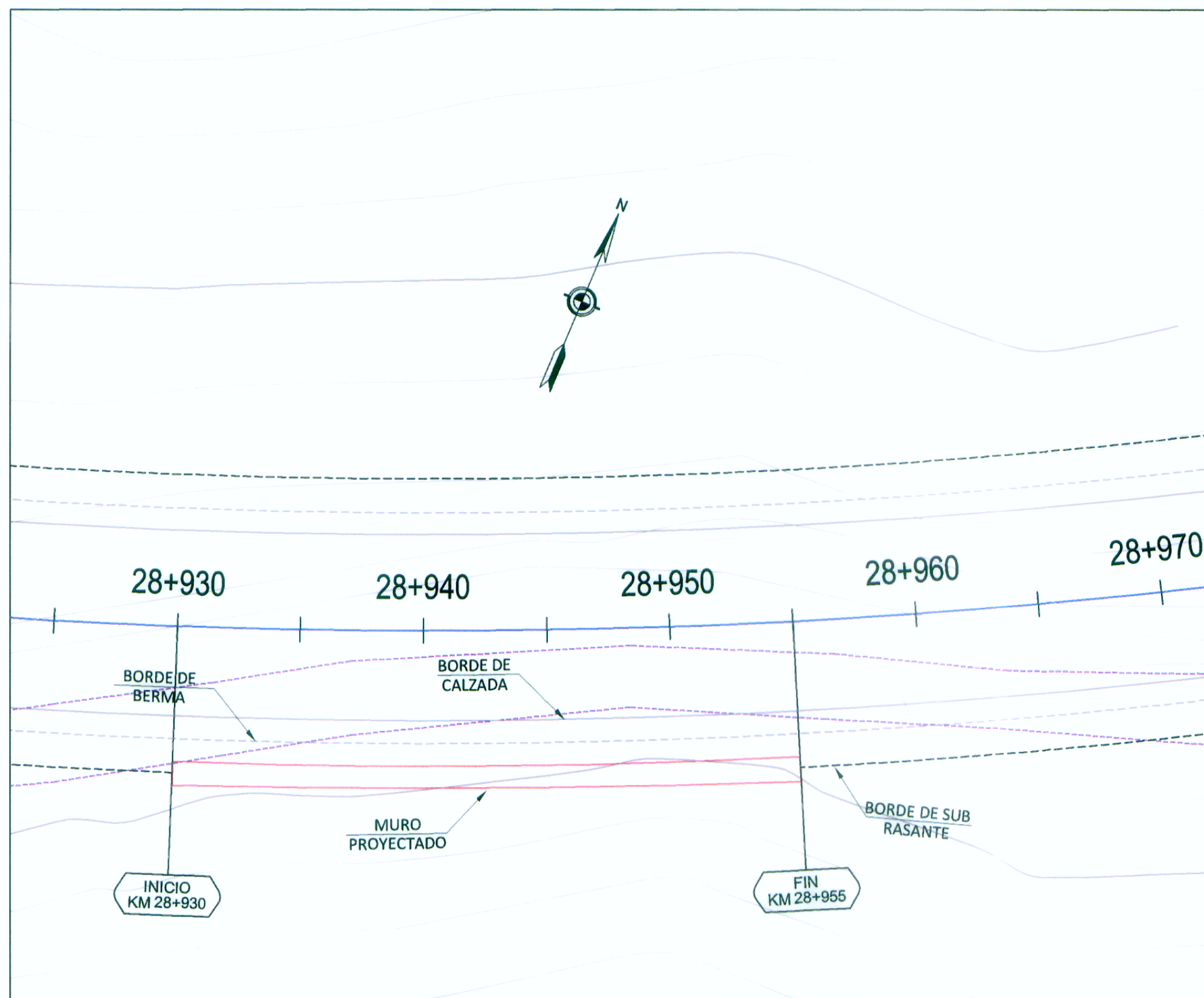
PLANTA
