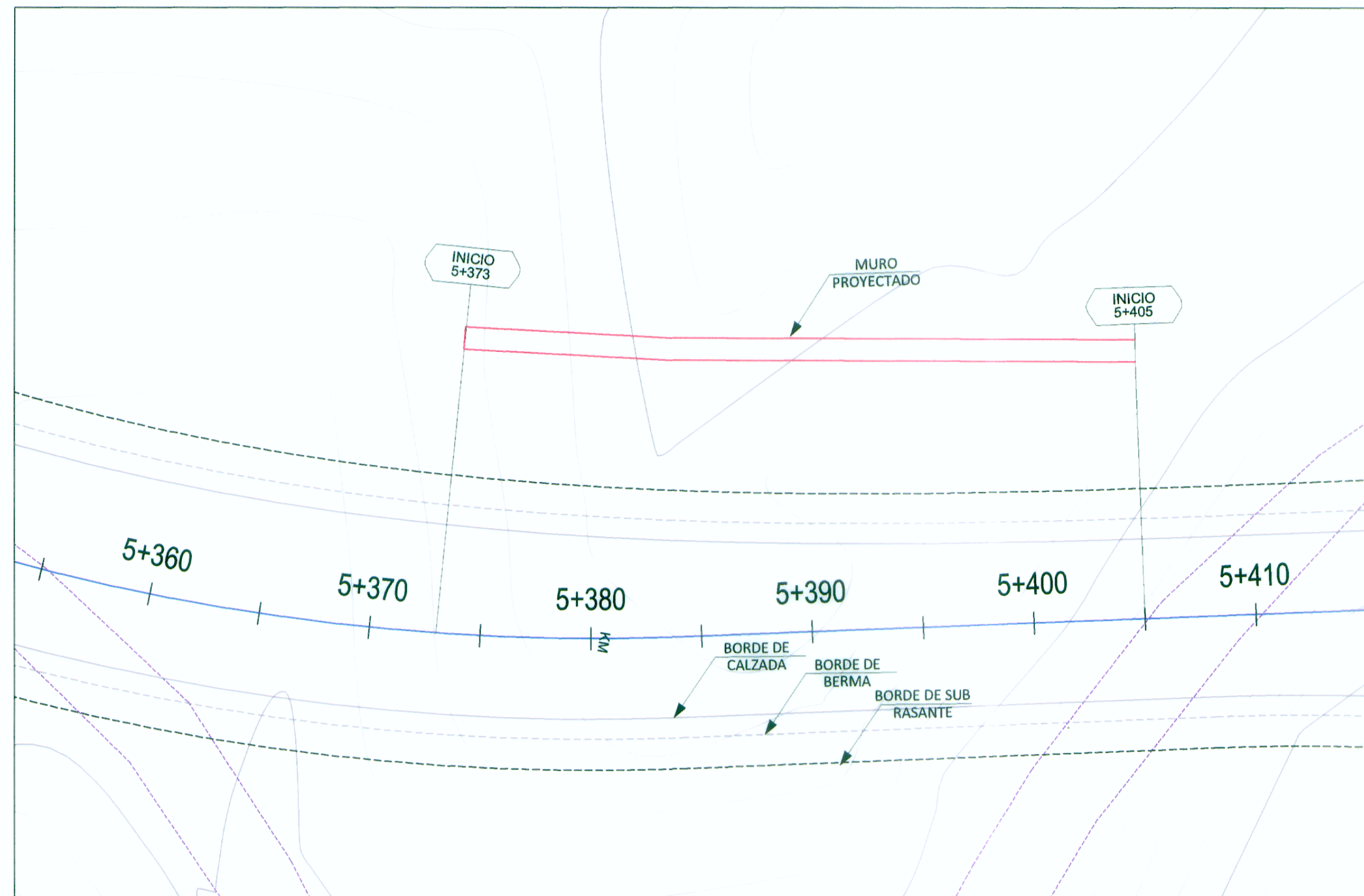
PLANTA
