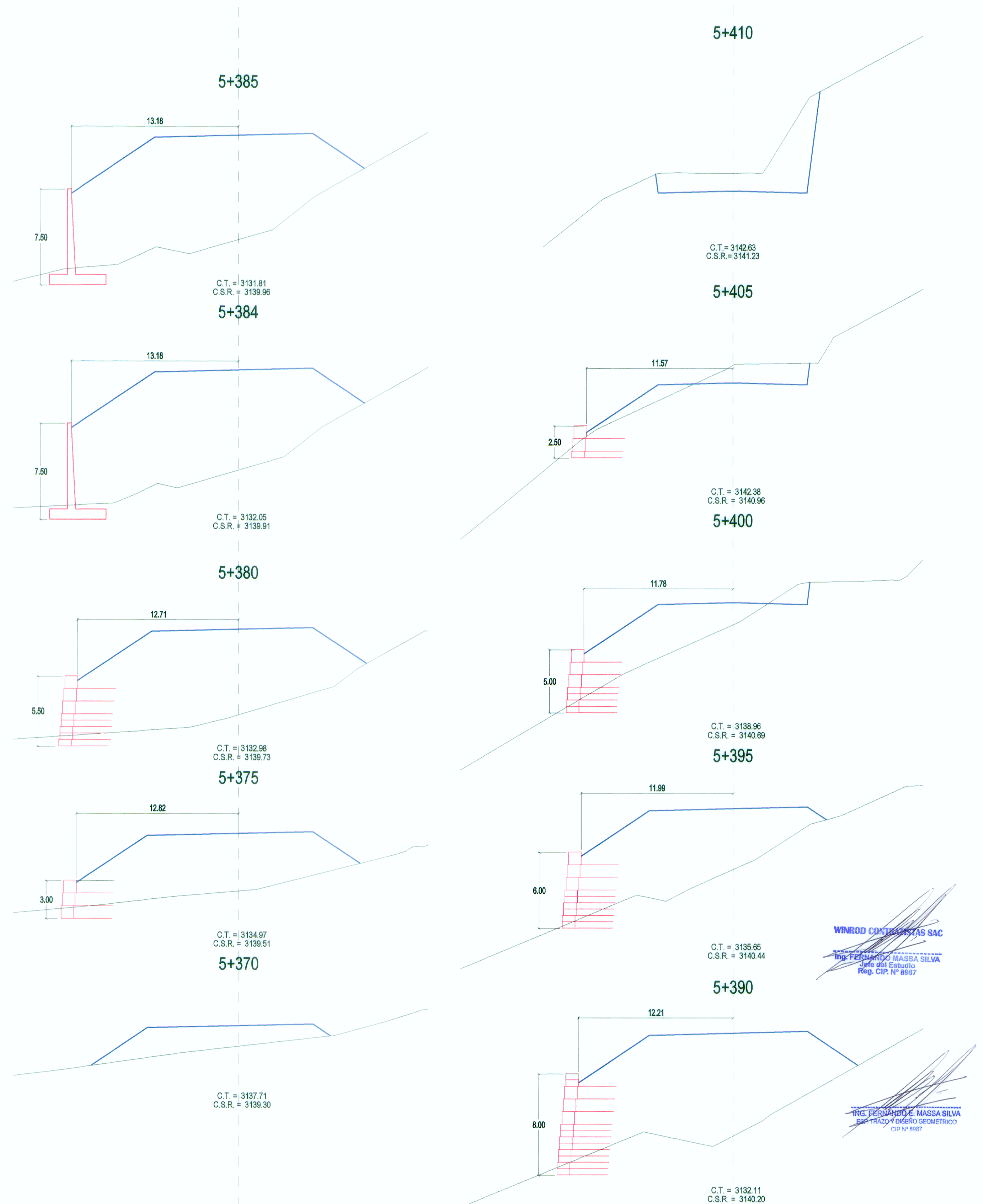
SECCIONES TRANSVERSALES
