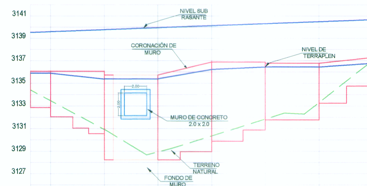
Muro 5+373 - 5+405
