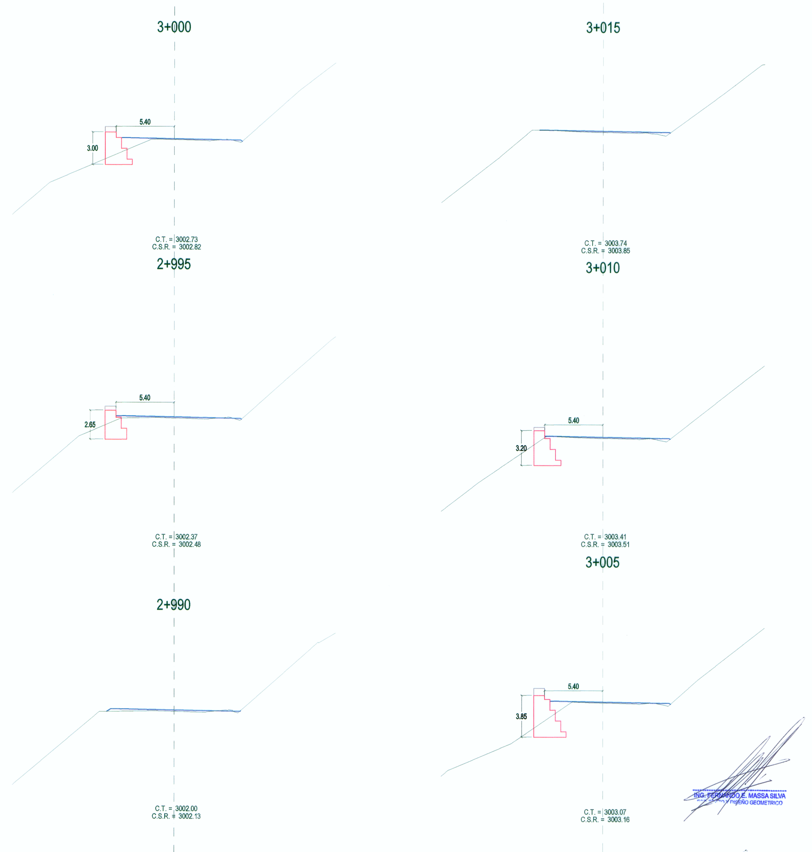
SECCIONES TRANSVERSALES
