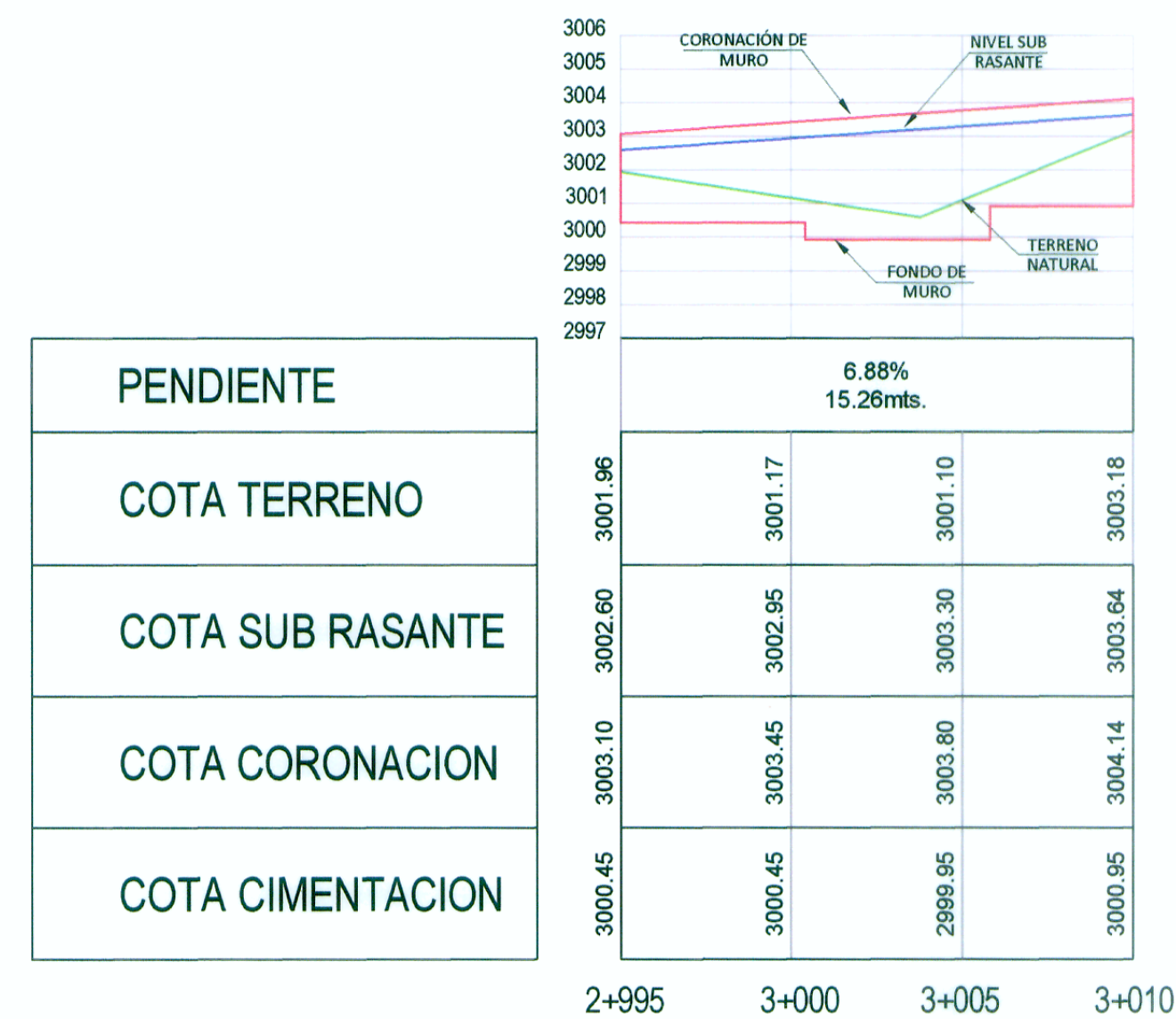
PERFIL LONGITUDINAL
