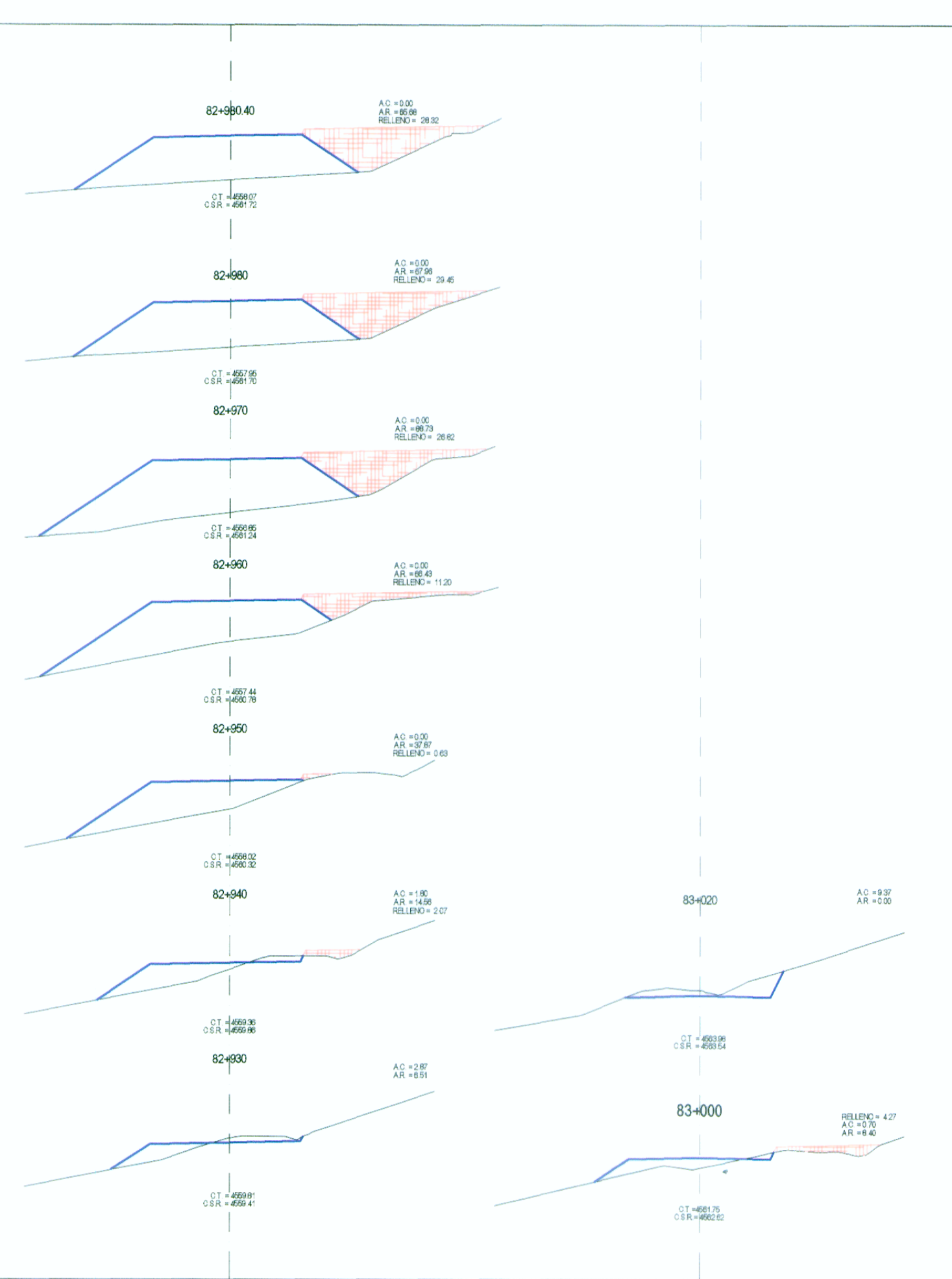
SECCIONES TRANSVERSALES ESCALA : 1/400
