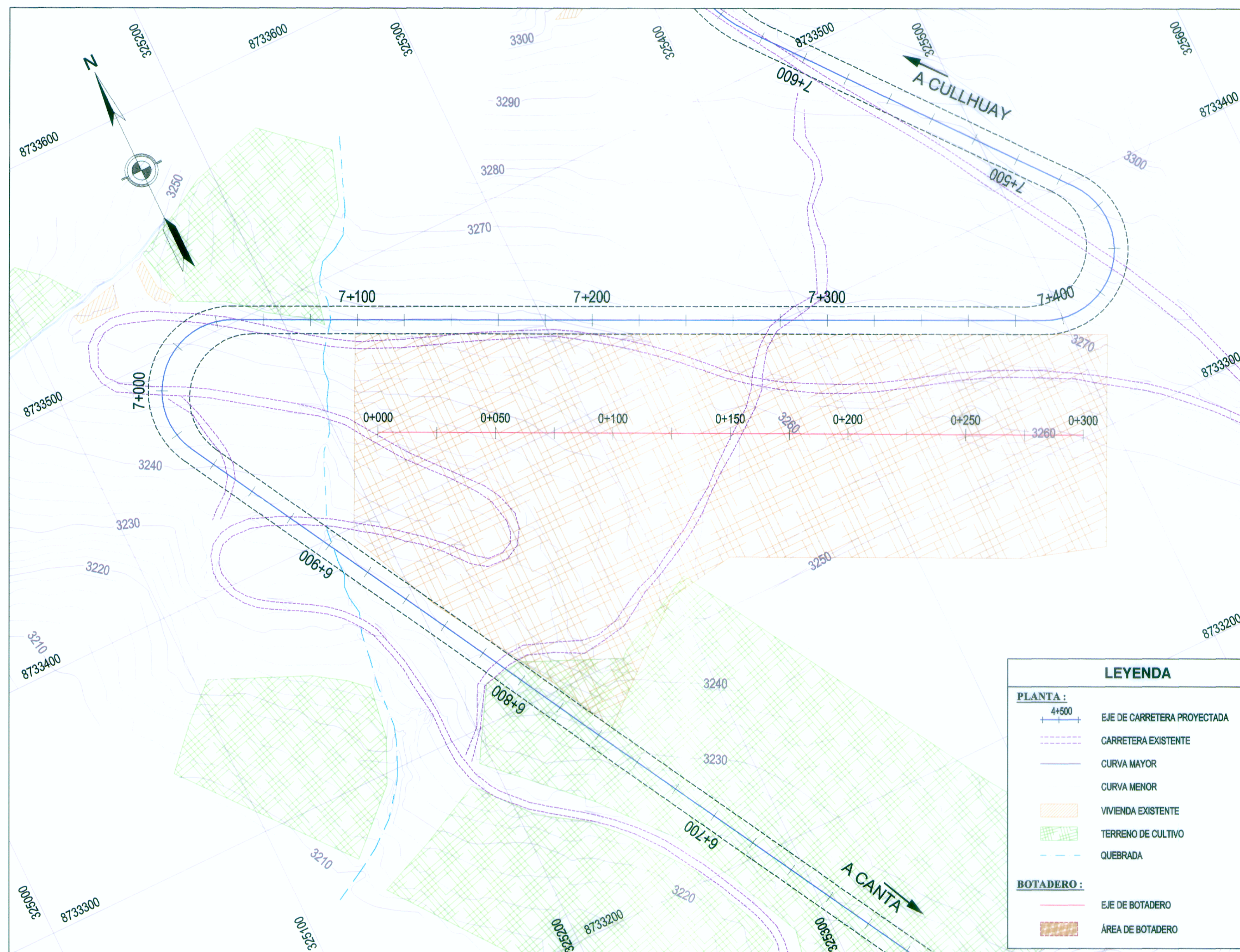
PLANTA ESCALA : 1/125
