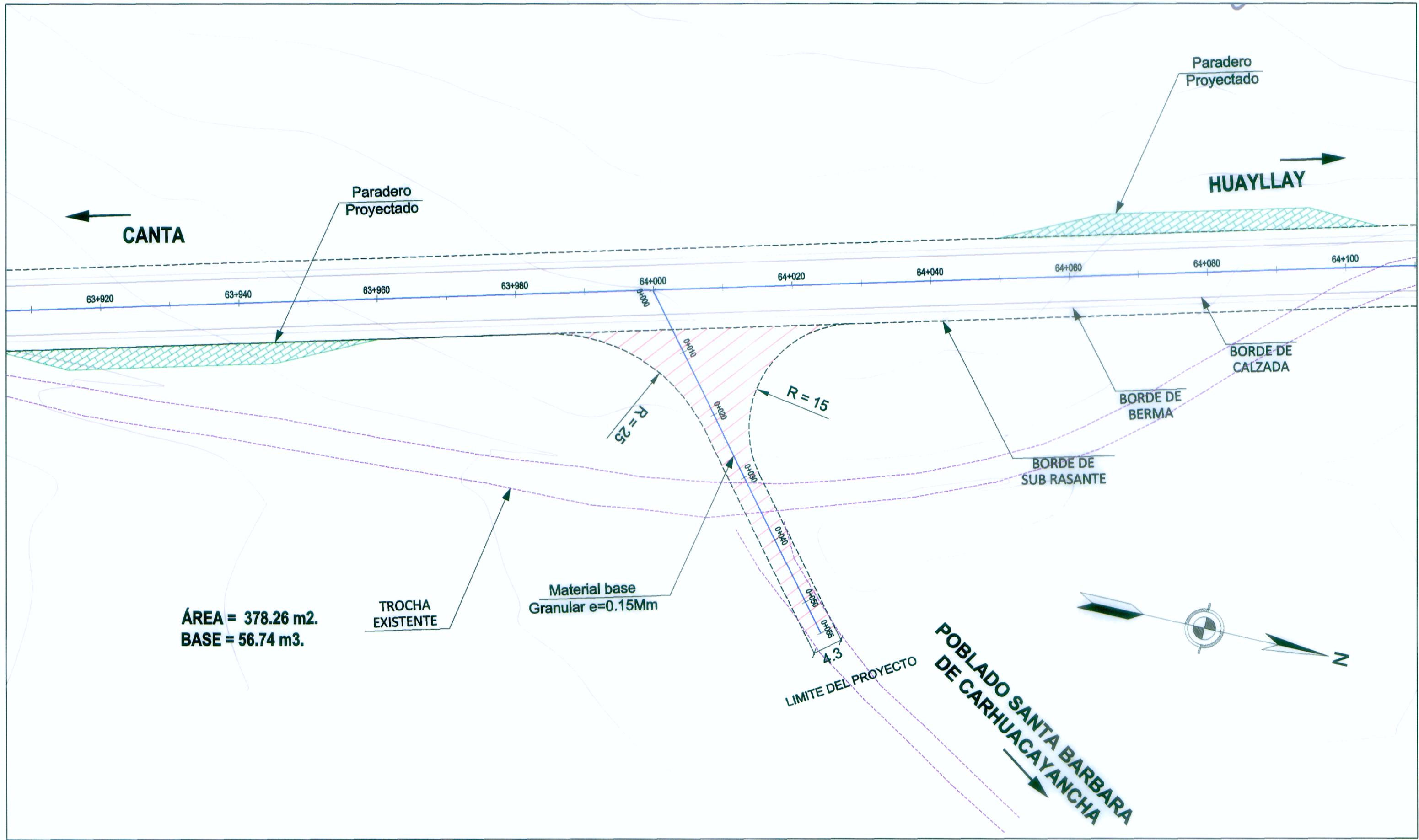
PLANTA ESC: 1/500
