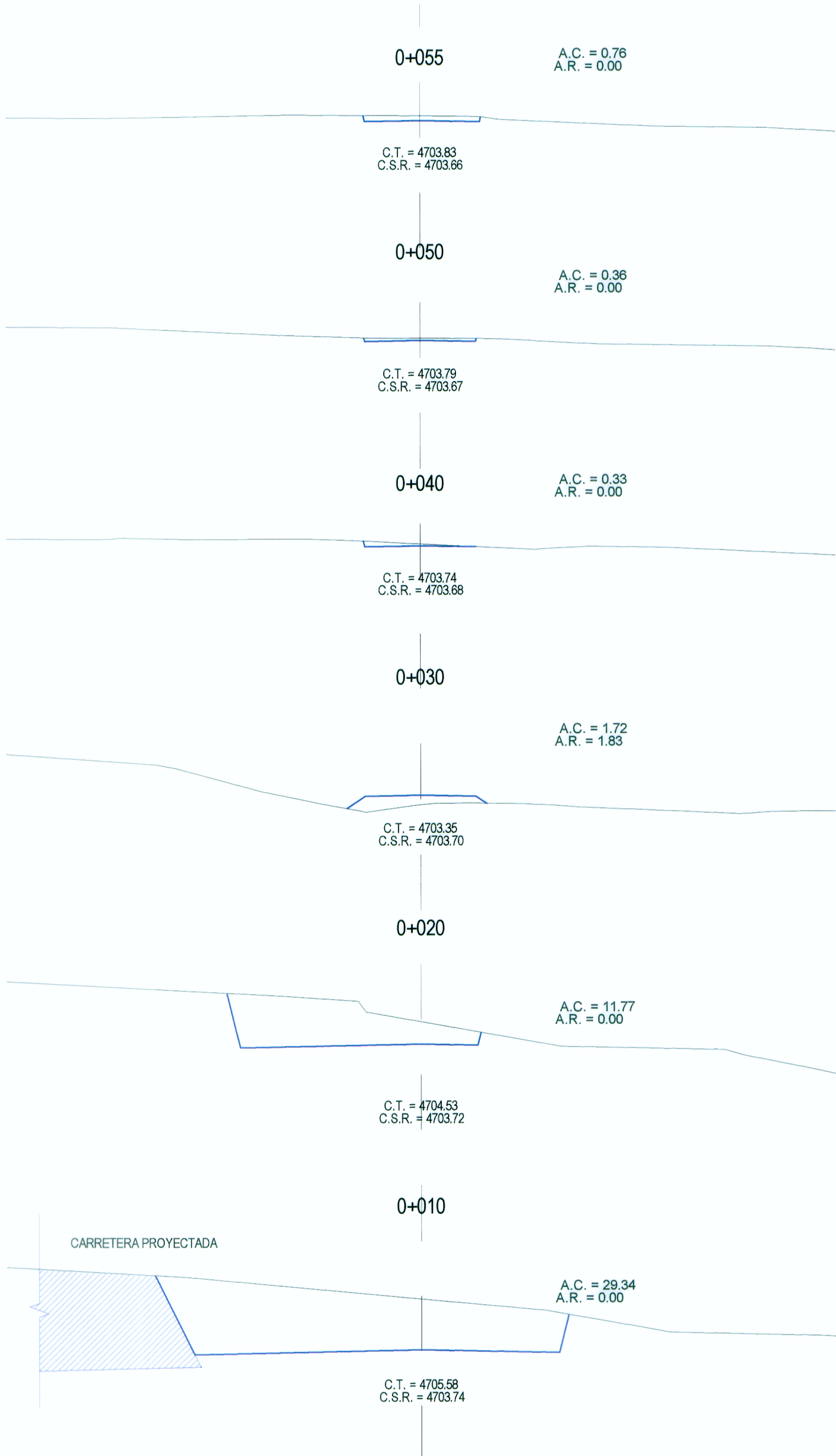
SECCIONES TRANSVERSALES ESC: 1/125
