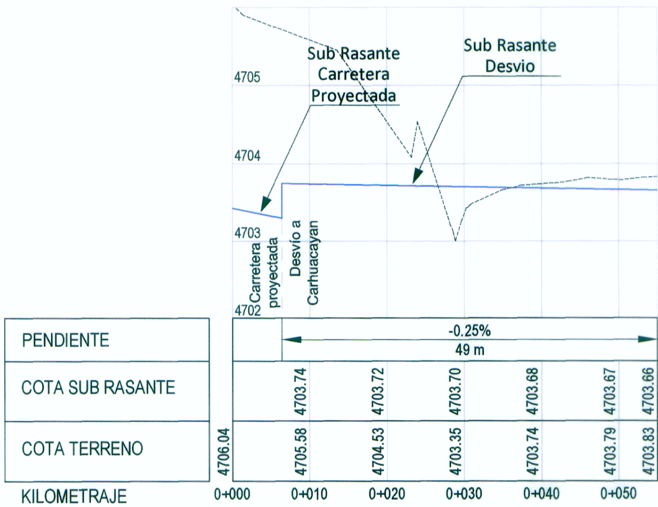
PERFIL LONGITUDINAL ESC: 1/500
