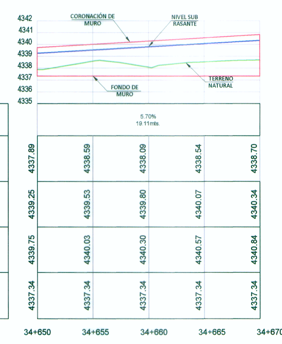
PERFIL LONGITUDINAL
