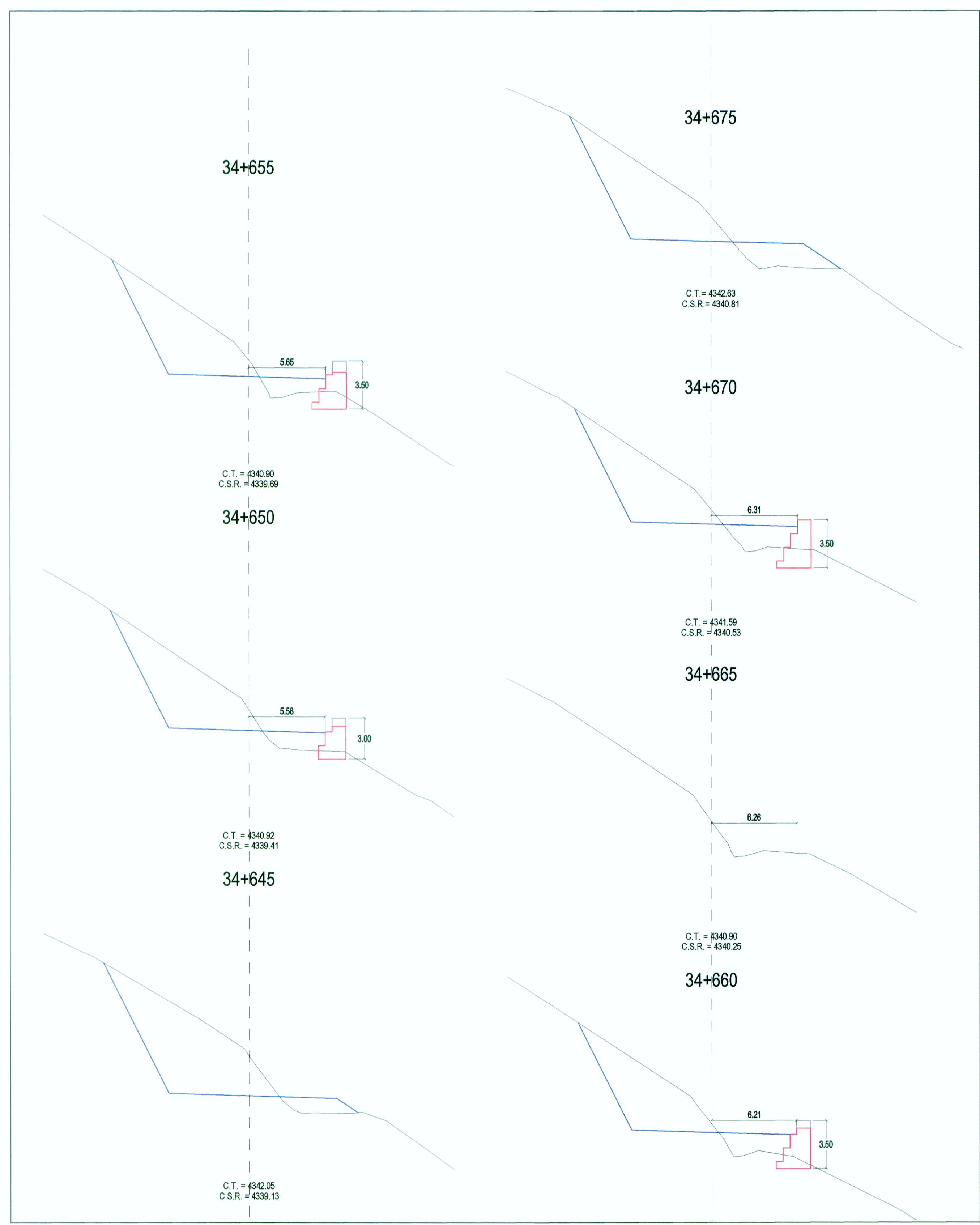
SECCIONES TRANSVERSALES
