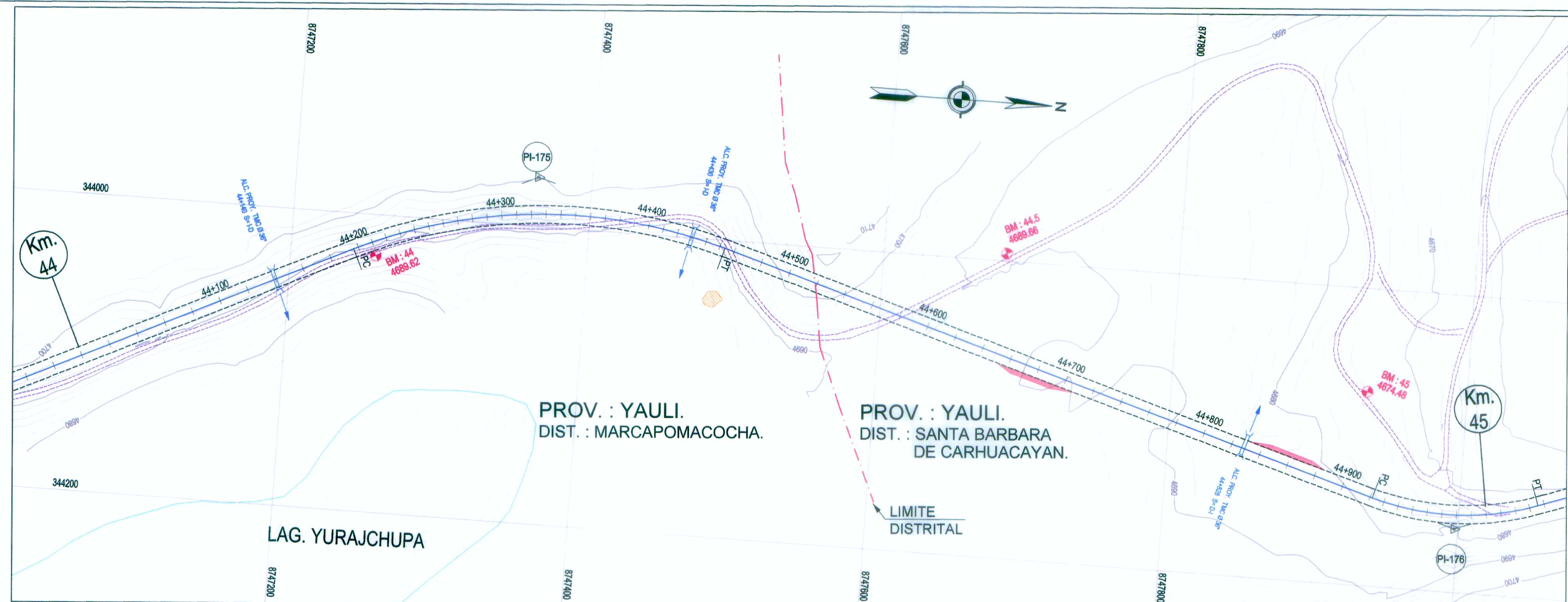
PLANTA
