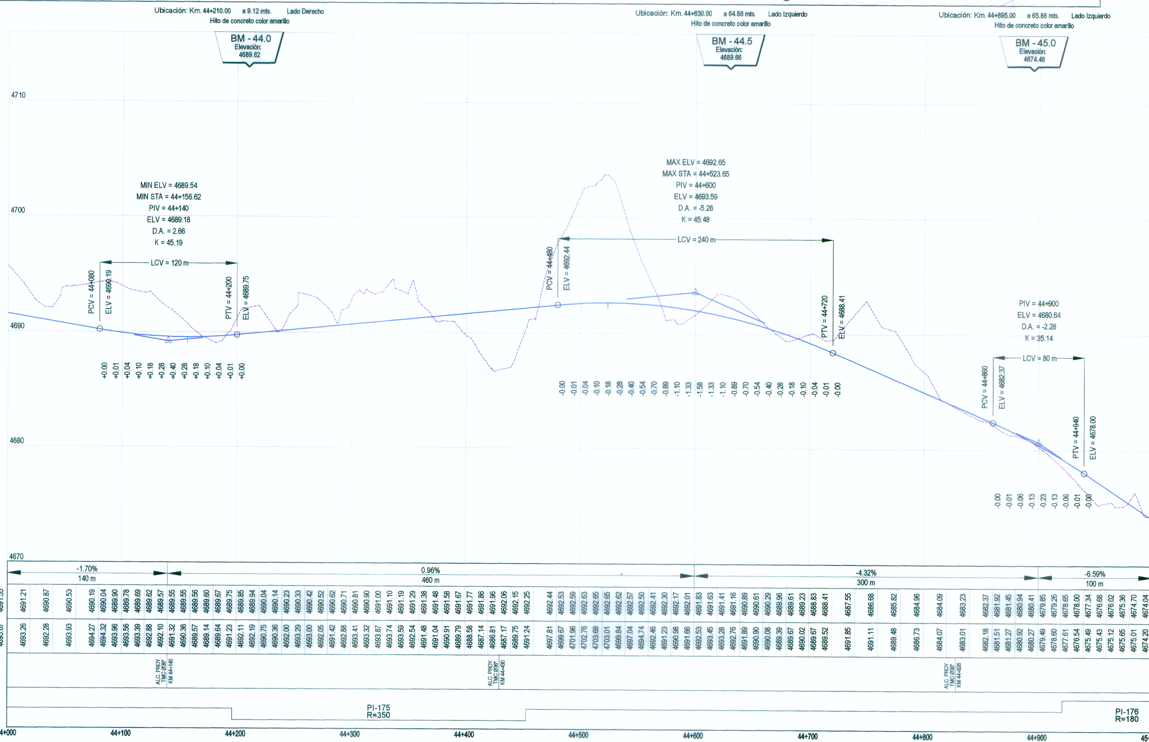
PERFIL LONGITUDINAL
