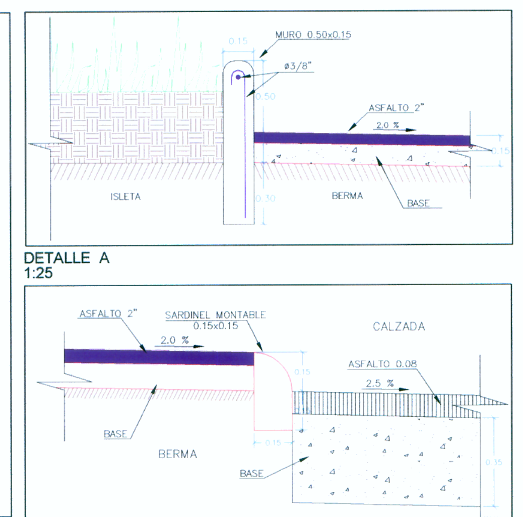
DETALLE B 1:20
